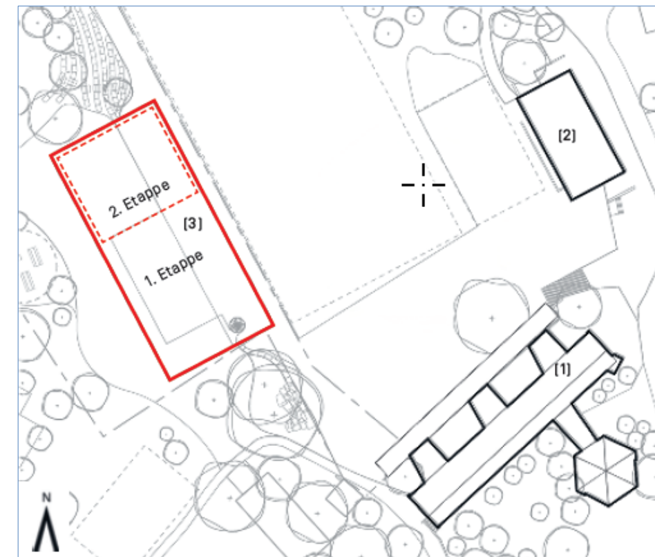
Abbildung: Situationsplan - Schulhaus Matt (1) | Turnhalle Matt (2) | Neubau (3)
