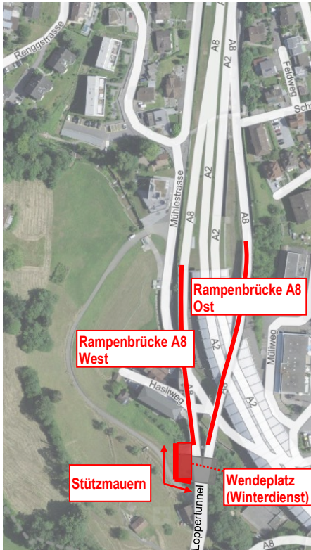
Rampenbrücken A8 und Stützmauern beim Wendeplatz Loppertunnel (Quelle: swisstopo)
